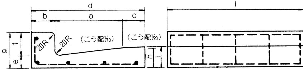
L 形側溝 1 種
