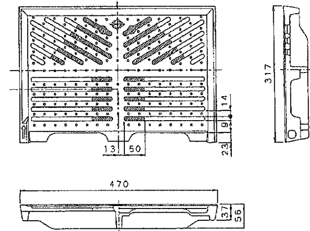
雨水枡蓋 タイプ2 (317×470)
